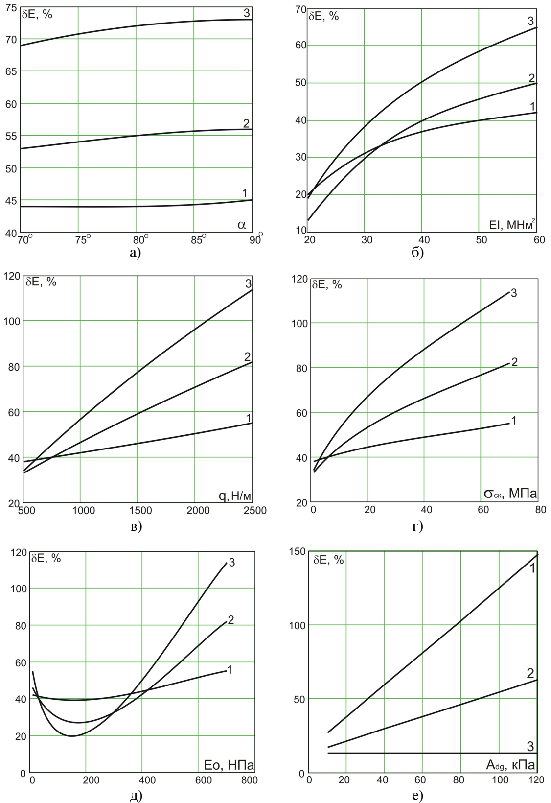
Рисунок 4 – Графічні залежності зміни величини \delta E для КНБК з різною кількістю ОЦЕ від техніко-технологічних і гірничо-геологічних умов буріння
