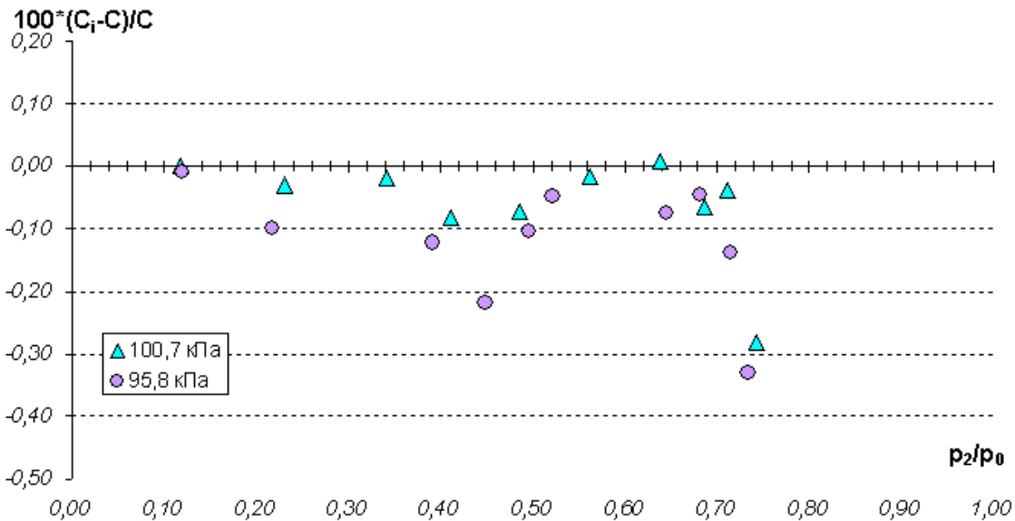
Рисунок 5 – Результати експериментальних досліджень тороїдального критичного сопла з діаметром горловини 1,2 мм
