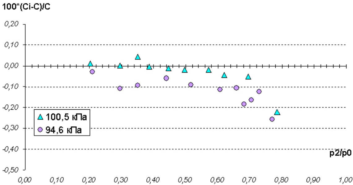
Рисунок 4 – Результати експериментальних досліджень тороїдального критичного сопла з діаметром горловини 1,9 мм
