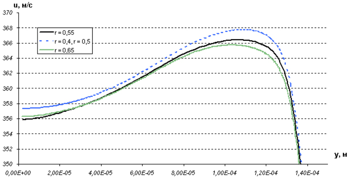
Рисунок 11 – Профіль швидкостей в перерізі переходу горловини сопла до дифузора за абсолютного тиску на вході сопла 101,325 кПа
