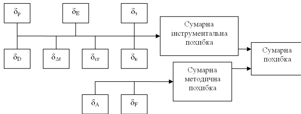
Рисунки 4 – Схема накопичення сумарної похибки вимірювального каналу тиску САК за відборами нафти з МН
