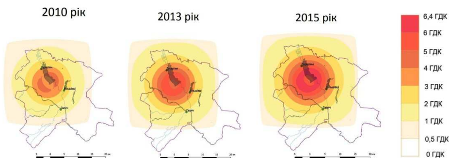
Рисунок 9 – Динаміка зміни концентрації групи сумарів у приземному шарі атмосфери
