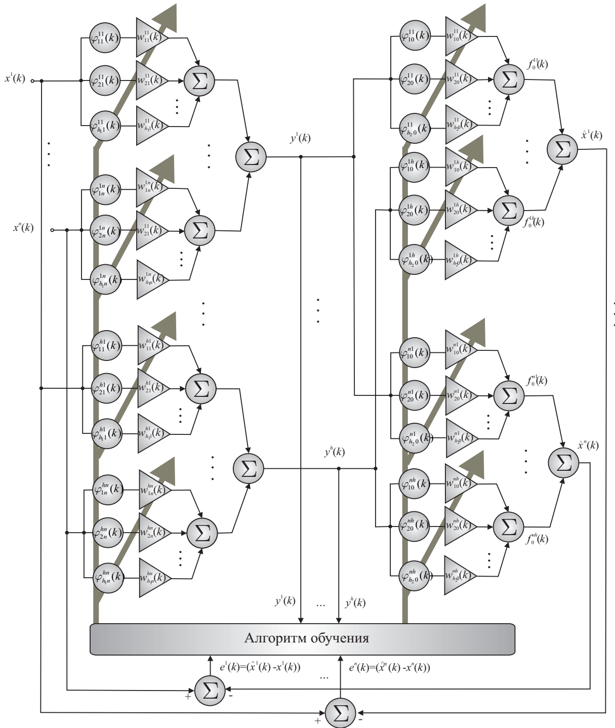
Рисунок 1 – Архитектура вэйвлет-нейро-компрессора
