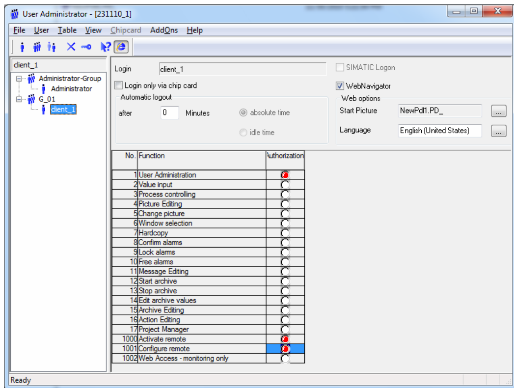
Рисунок 5 – Вікно створення груп і окремих користувачів з відповідними правами доступу в програмному модулі User Administrator SCADA WinCC
