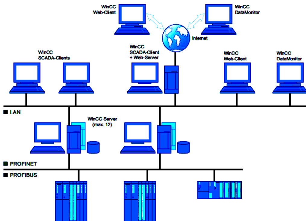
Рисунок 2 – Функціональна схема WEB-орієнтованої розподіленої клієнт-серверної системи управління на базі SCADA WinCC з опційним програмним модулем WinCC Web-Navigator
