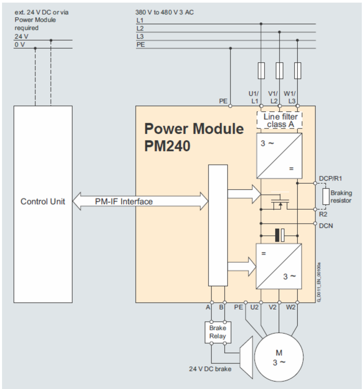
Рисунок 8 – Функціональна схема і комунікаційні з'єднання силового модуля PM240 системи частотного управління електроприводом Sinamics G120
