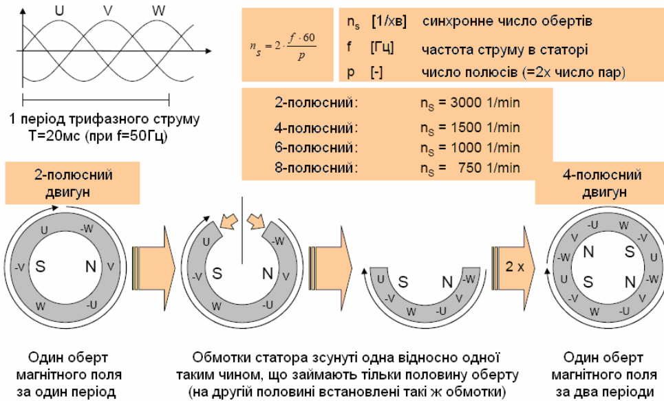
Рисуюнок 1 – Електрична будова і розрахункові вирази для асинхронного електропривода
