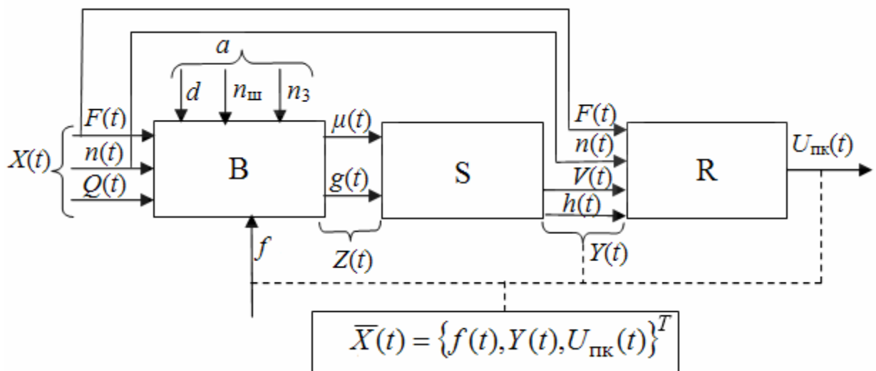
Рисунок 1 – Структурна схема процесу буріння свердловин як об'єкта контролю буримості в просторових координатах ( \bar{X}_k(t) – контрольовані параметри)
