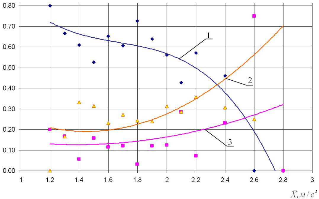
1 – бездефектний стан; 2 – руйнування бабітового шару; 3 – збільшений зазор
