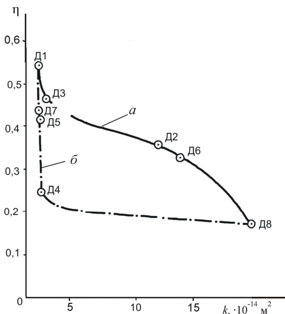
Рисунок 2 – Залежність кінцевого коефіцієнта нафтовилучення \eta від коефіцієнта загальної проникності k моделі тріщинувато-пористого пласта за різних ступенів тампонування тріщини відповідно номерам дослідів для випадків тампонування зі сторони відбирання (а) і зі сторони нагнітання (б)
