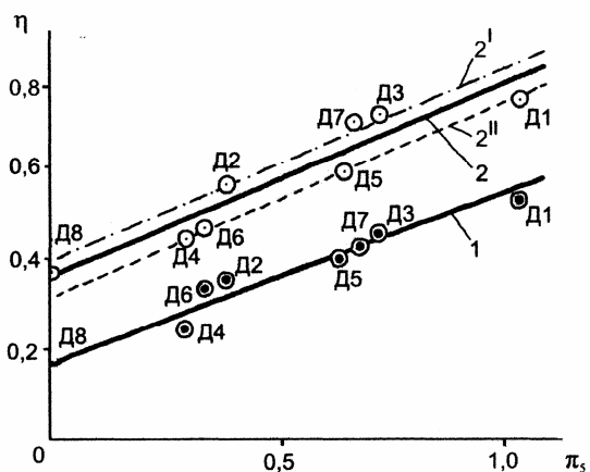
Рисунок 1 – Залежності коефіцієнтів \eta безводного нафтовилучення (1) і кінцевого нафтовилучення (2) від ступеня тампонування тріщини (параметра \pi_3 ) за простяганням у випадку розміщення тампона відповідно зі сторони відбирання (2') і нагнітання (2'')
